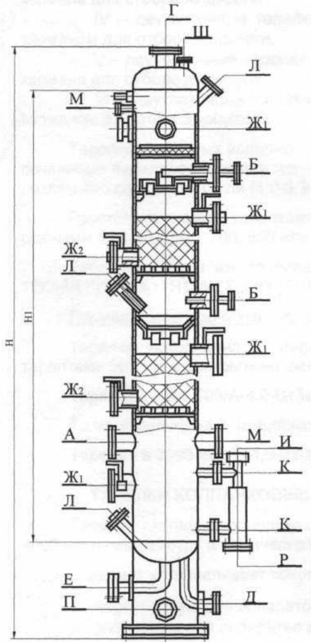
Рис. 5.4 Колонные аппараты с насыпной насадкой цельносварные диаметром от 1000 до 2800 мм черт. 154-3536.00.000 ВО
