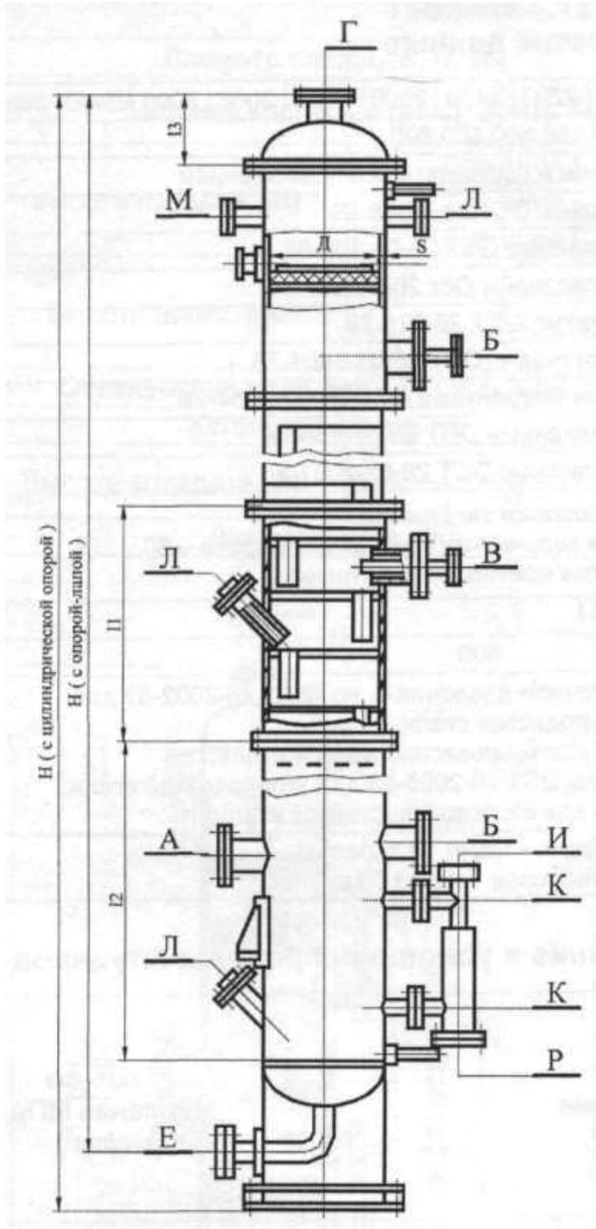
Рис. 5.1 Колонные аппараты тарельчатые царговые 0 от 400 до 800 мм черт. 153-3537.00.000 ВО.
